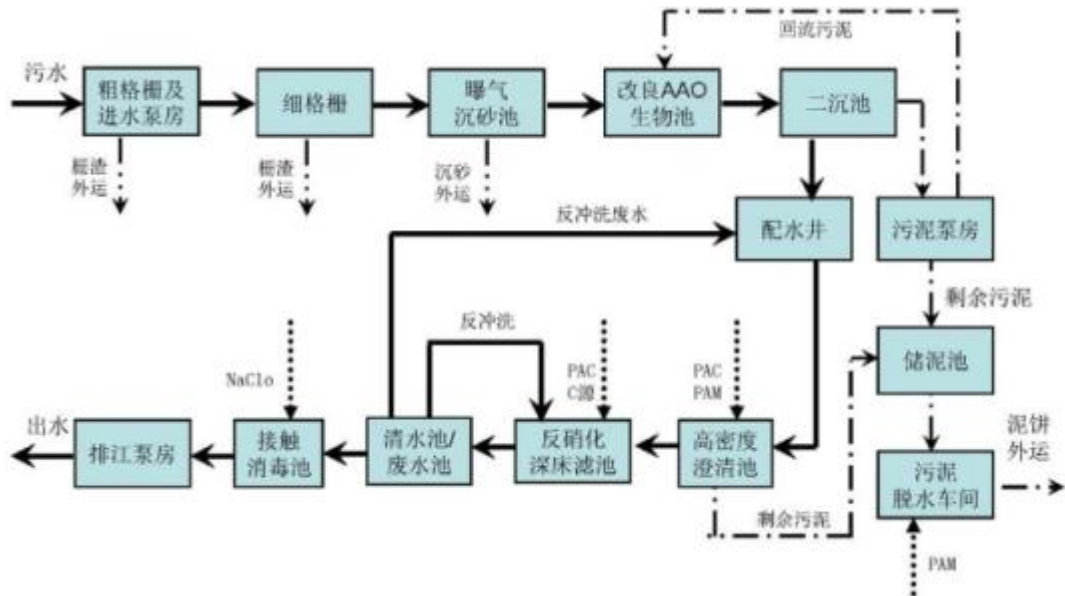
图 4-2 芜湖市湾沚区新芜开发区城东污水处理厂废水处理工艺
