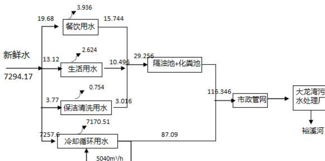
图 2-2 本项目水平衡图 (m 3 /d)
