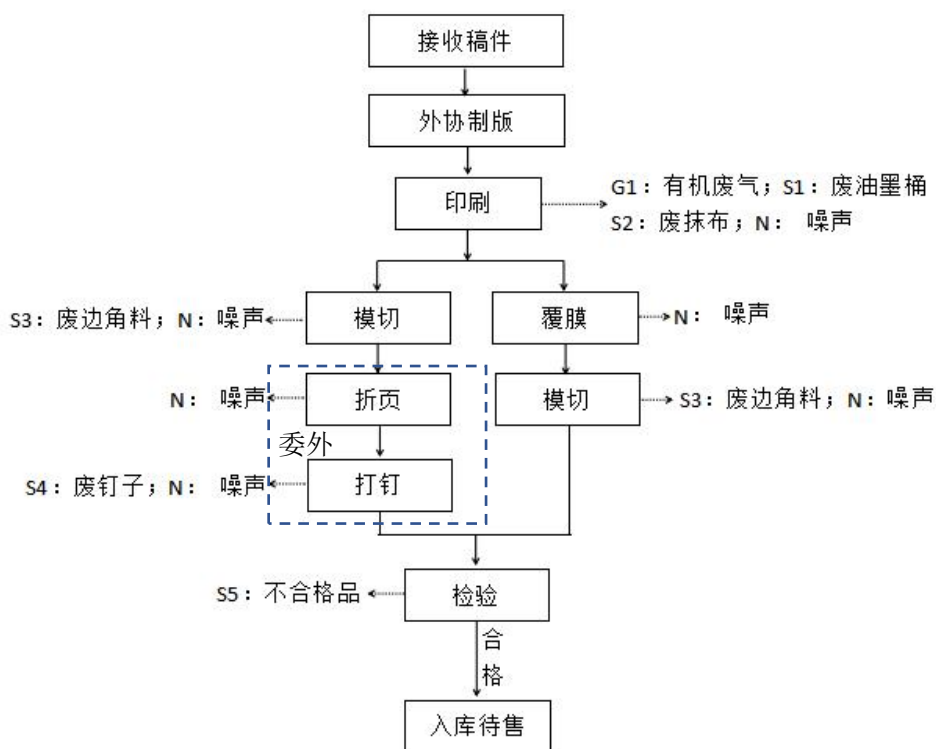
图 2-1 生产工艺及产污节点图
